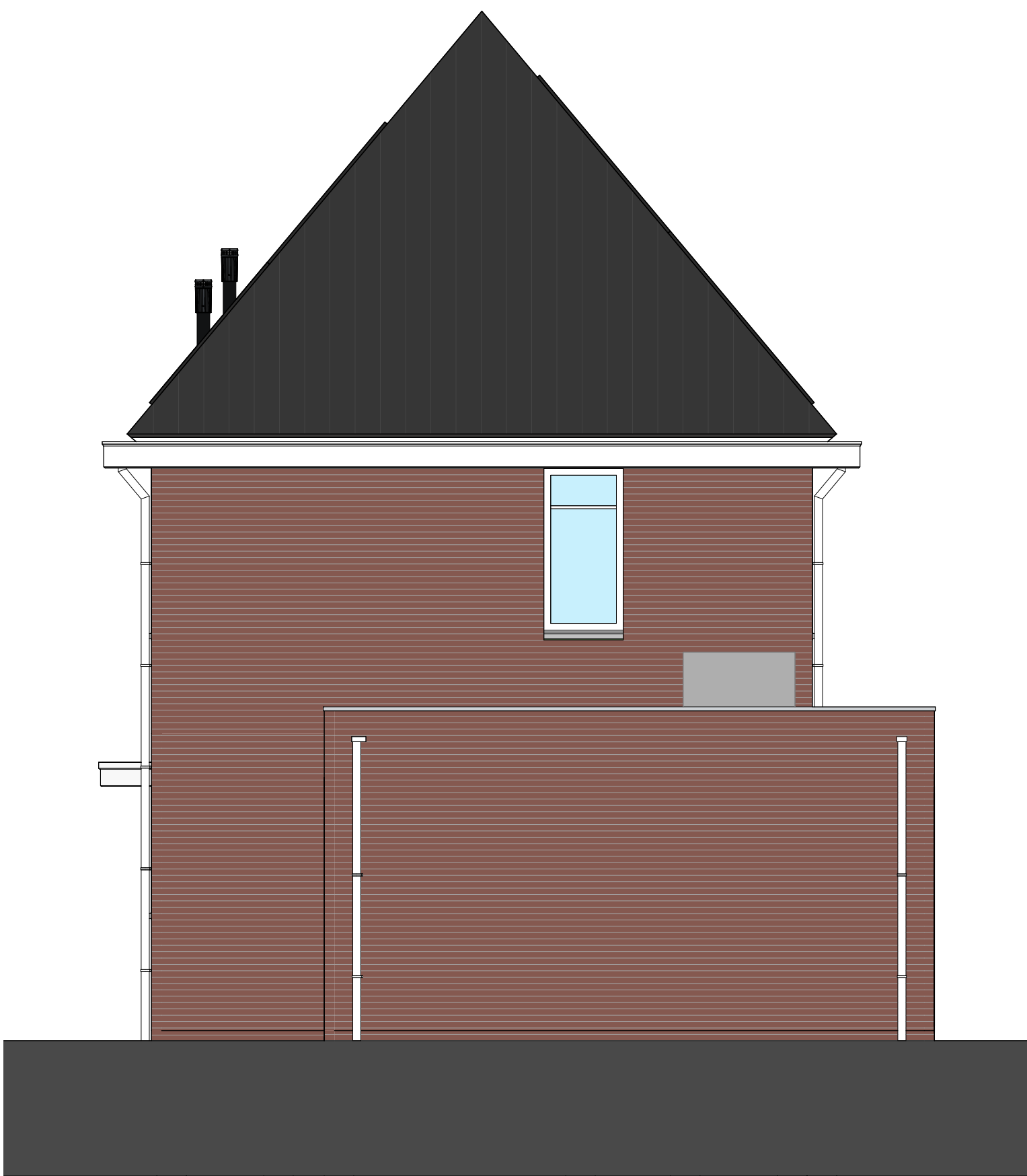
Rechter zijgevel 1 : 50
